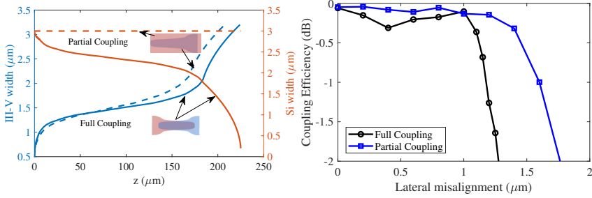
Figuur 3: (links) De III-V en Si adiabatische koppelstructuur in de lengterichting. De blauwe lijn en de linker verticale as stellen de III-V adiabatische conische vorm voor de gedeeltelijke en volledige koppelingsontwerpen. De rode lijn en de rechter verticale as representeren de adiabatische conische vorm van Si en de breedte van de Si golfgeleider in het geval van respectievelijk volledige koppeling en gedeeltelijke koppeling; (rechts) De gesimuleerde koppelingsefficiëntie van de adiabatische structuren voor de ontwerpen voor gedeeltelijke en volledige koppeling versus de laterale uitlijning.
