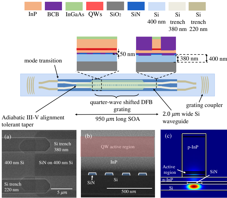
Figuur 6: Schematische voorstelling van het ontwerp van de DFB-laser met aanzicht in dwarsdoorsnede van de adiabatische structuur en het zijaanzicht van het DFB-rooster. SEM-afbeeldingen van a) overgang tussen DFB sectie en passieve siliciumgolfgeleider, b) longitudinale dwarsdoorsnede van het DFB-rooster en c) het modeprofiel in de versterkingssectie.
