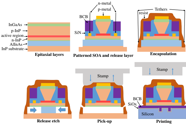
Figuur 1: Schematische voorstelling van het micro-transfer-printproces van geprefabriceerde SOA-coupons.
