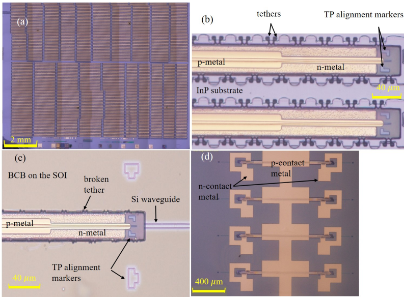
Figuur 2: Microscoopbeeld van a) verwerkte SOA-coupons op het InP-substraat, b) twee SOA-coupons van (a) waarop wordt ingezoomd, c) geprinte SOA-coupon op een Si-golfgeleider, en d) III-V-on-Si SOA's met metaalcontacten.
