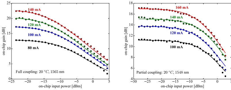
Figuur 5: Variatie van de versterking op de chip met het ingangsvermogen op de chip voor verschillende instelstromen, (links) voor het ontwerp met volledige koppeling bij 1565 nm, (rechts) voor het ontwerp met de gedeeltelijke koppeling bij 1548 nm.
