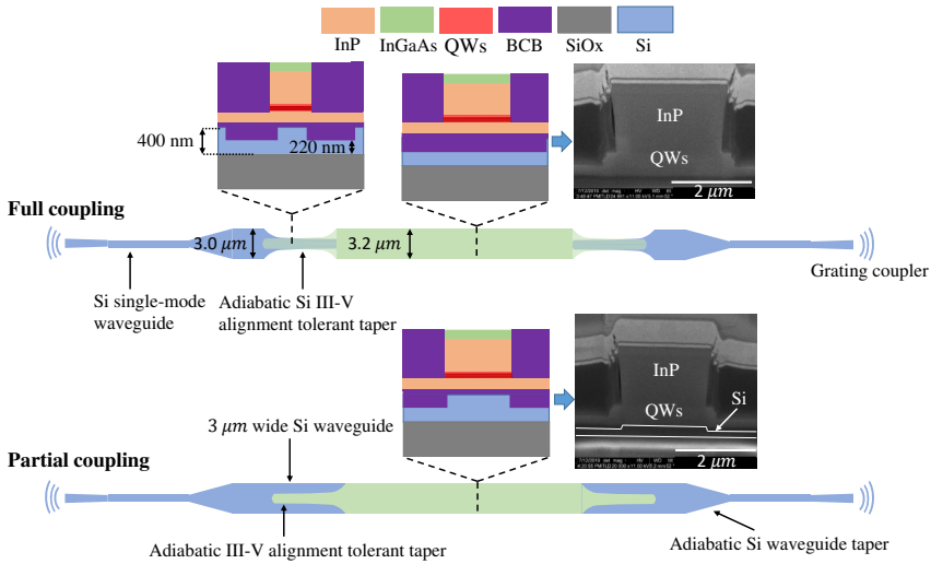
Figuur 4: Schema's en FIB-doorsneden die het ontwerp van de volledige koppeling en gedeeltelijke koppeling voor III-V-op-Si SOA's illustreren.
