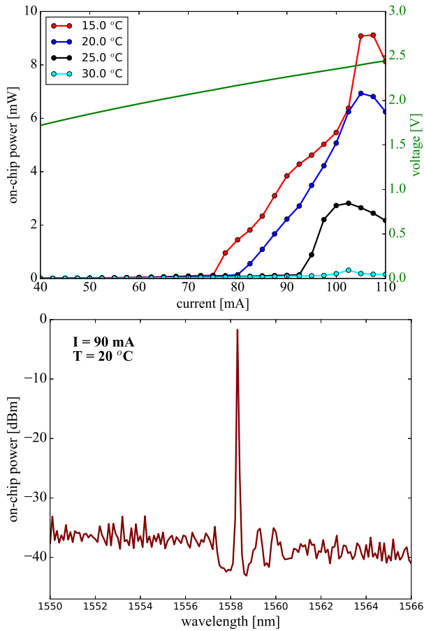
Figuur 7: (boven) Golfgeleider-gekoppeld uitgangsvermogen (enkel-zijdig) als functie van stroom voor verschillende bedrijfstemperaturen en de stroom-spanningskarakteristiek, (onder) Gemeten spectrum (0,05 nm resolutie) bij 90 mA en 20 °C bedrijfstemperatuur.
